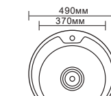
L74949-6 Ø 490x170 Врезная
