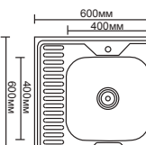
L96060-6L L96060-6R 600x600x170 Накладная
