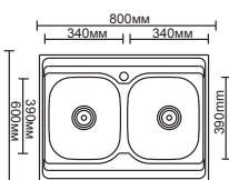
L98060B-6 800x600x170 Накладная
