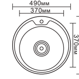
L64949-6 Ø 490x170 Врезная
